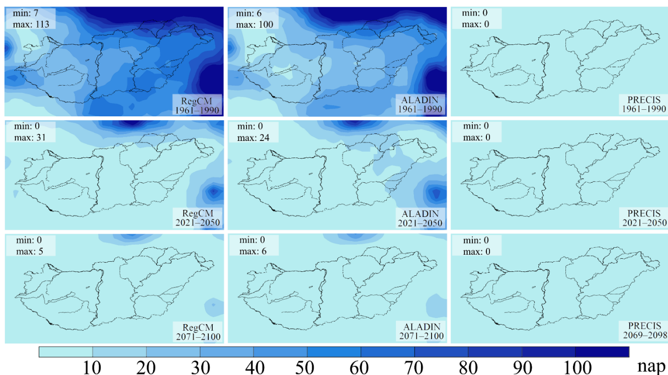
F10. ábra: A -17\text{ °C} alatti minimumhőmérsékletű napok száma a nyugalmi időszakban ( DN_{B17m_D}^g , nap) Magyarországon az '5mid' módszer alapján. A sorok a három vizsgált időszakot mutatják: 1961–1990 (fent), 2021–2050 (középen), és 2071–2100 68 (lent). Az oszlopokban a három különböző modell eredménye látható: RegCM (balra), ALADIN (középen), és PRECIS (jobbra).
