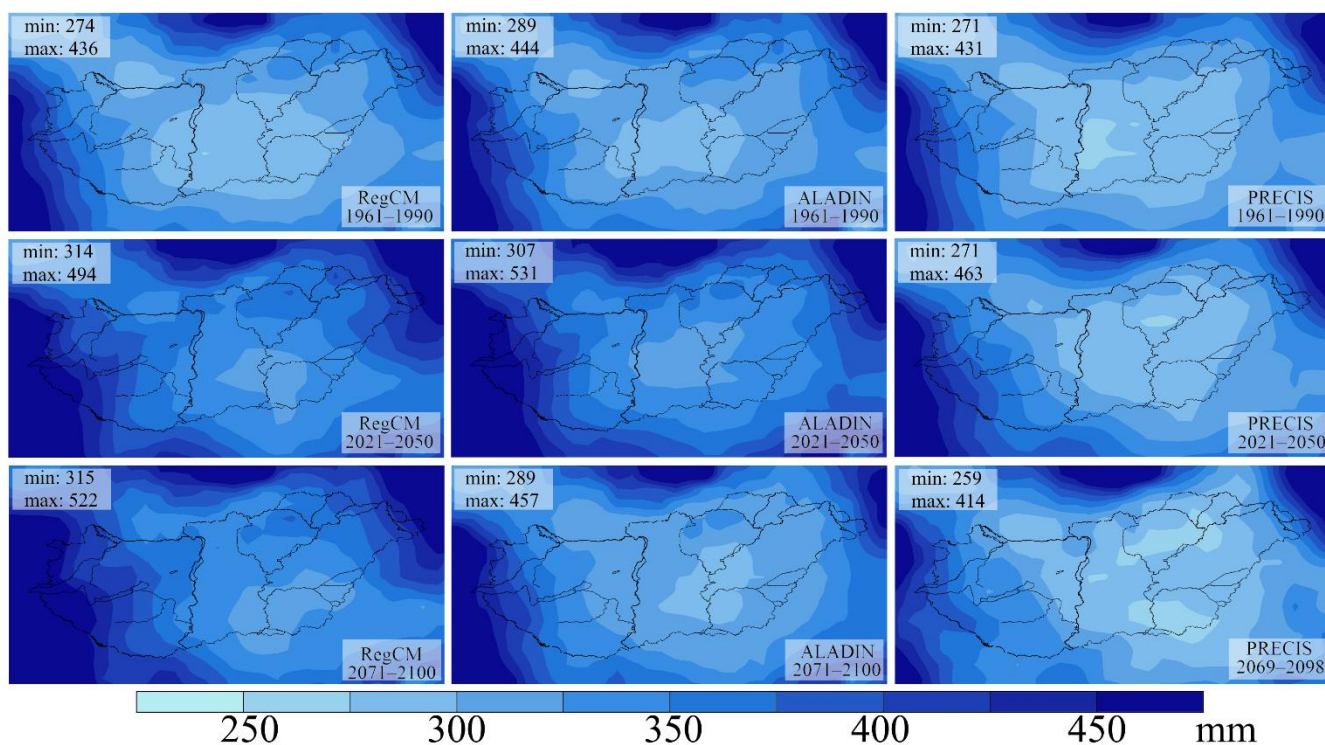
12. ábra: Az átlagos vegetációs időszaki csapadékösszeg ( P_{GS}^g , mm) Magyarországon az ‘5mid’ módszer alapján. A sorok a három vizsgált időszakot mutatják: 1961–1990 (fent), 2021–2050 (középen), és 2071–2100 39 (lent). Az oszlopokban a három különböző modell eredménye látható: RegCM (balra), ALADIN (középen), és PRECIS (jobbra).
